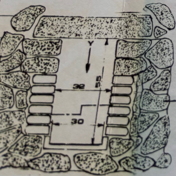
Coupe du tronçon d' Aqueduc découvert à Eclaiibes LE GRAND AQUEDEC DE BAWY H BEY VELEET, 1962
